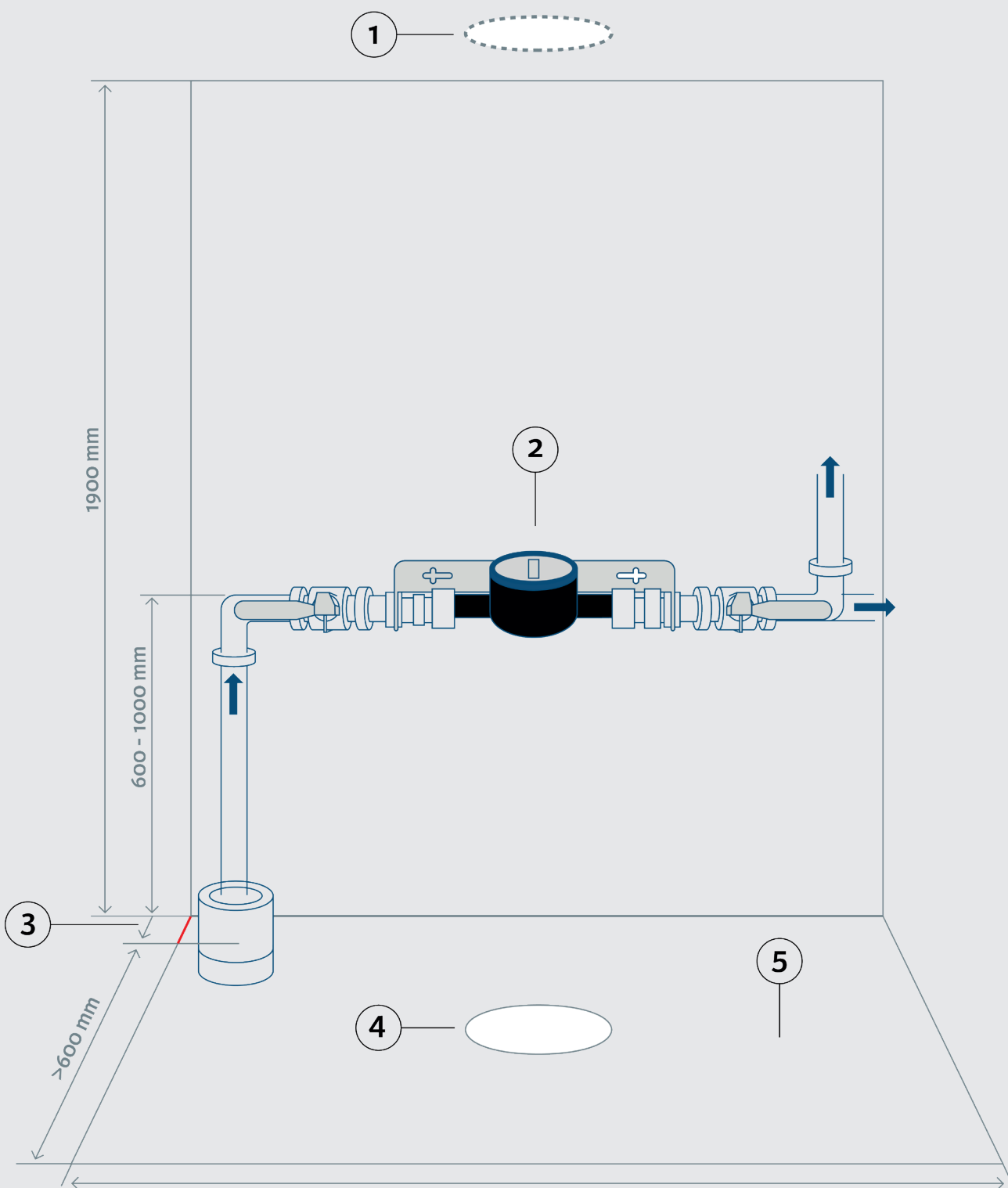
Mätarplats med utrymmesbehov för en mätare för hushållsbehov, enligt Svenskt vattens publikation för vattenmätare
