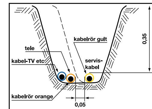
Figur 2. Utförande av kabelgrav visande samförläggning av el- och teleservis på tomtmark.
